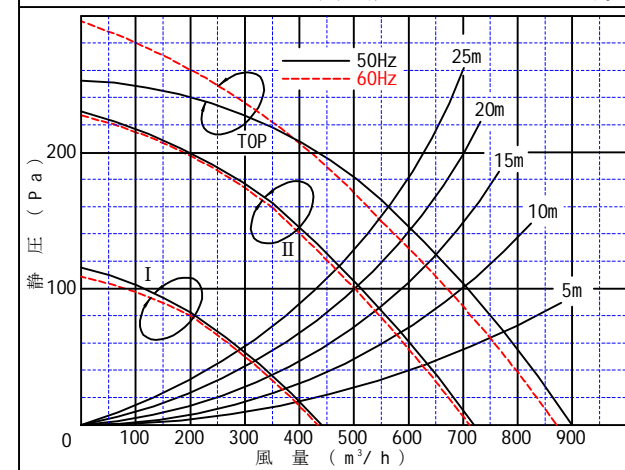
静圧・風量曲線 ※抵抗曲線はφ150スパイラルダクトを示す。
